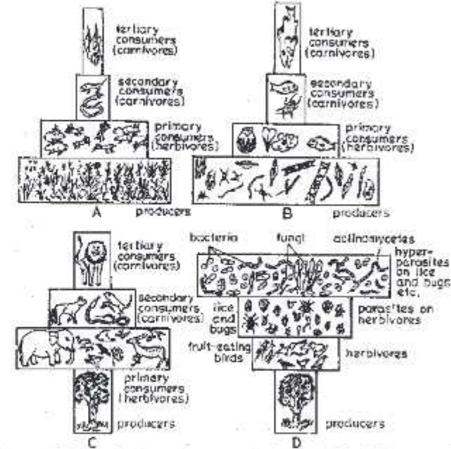
आकृती ३.७ : विविध प्रकारच्या परिसंस्था/अन्न साखळ्यांमधील संख्याविनिमय अ-गवताळ परिसंस्था, ब-तलाव परिसंस्था, क-जंगल परिसंस्था, ड-सिजीवी अन्न साखळी. अ त क मध्य सिजीवी सूक्ष्मजीव व जमीनीतील प्राणी घेतिलेले नाहीत.
