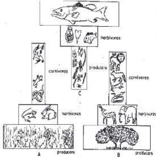
आकृती ३.८ : अ-क वगैरेच्या पिरसंस्थामधील जैववस्तुमानाचा मनोरा (gdry wt./unit area) अ-गवताळ पिरसंस्था, ब-जंगल पिरसंस्था, क-तलाव पिरसंस्था
